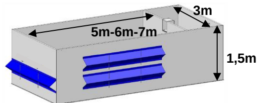
TfN15/18/21 mit 2 Versteigungsblechen bei bündige oder normalen +10cm bis 15cm Einbau
