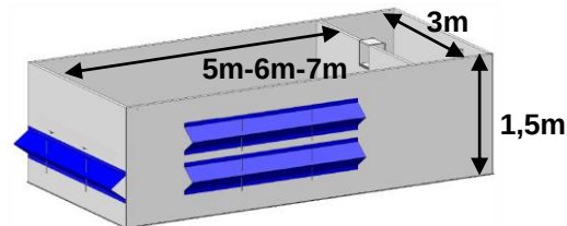
TfN15/18/21 mit 2 Versteifungsblechen bei bündiger oder normalen +10cm bis 15cm Einbau
