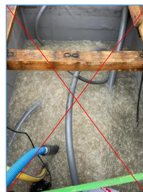
Skimmerteich bei Bubblen nach ca. 90 Tagen. (Wasser ist trüb, da zu spät rückgespült).
