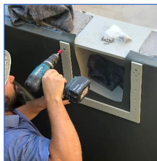
Skimmerklappen Flansch befestigen.
